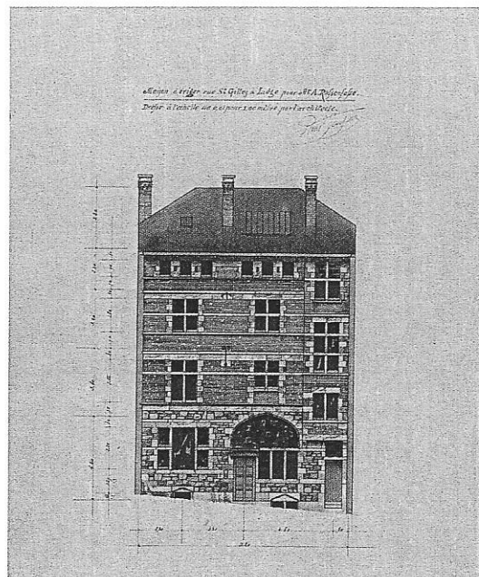
Maison Rassenfosse, rue Saint-Gilles, 1898 © Centre d'Archives et de Documentation de la C.R.M.S.F., Liège - fonds Paul Jaspar, dépôt de la Ville de Liège
